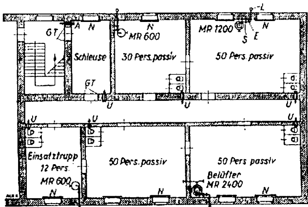
A - Abluftventil E - Entwässerung L - Luftansaugleitung GT - gasdichte Tür N - Notausstieg S - Absperfschieber (Gußrohr oder Innrohr) U - Überdruckventil
